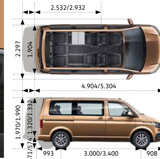
Abmessungen in mm 4) (kurzer/ langer Radstand)
